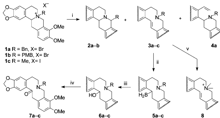
Scheme 3. Synthesis of protopines: i) HNa/benzene/DMSO, room temp.; ii) BH 3 ·THF, room temp.; iii) H 2 O 2 /phosphate buffer (pH = 8)/THF, reflux; iv) PCC/CH 2 Cl 2 /NaAcO, room temp.; v) MeI/CHCl 3 , room temp.
